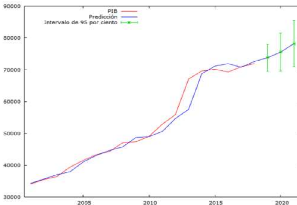
Fig. 10. Predicciones de la variable PIB
