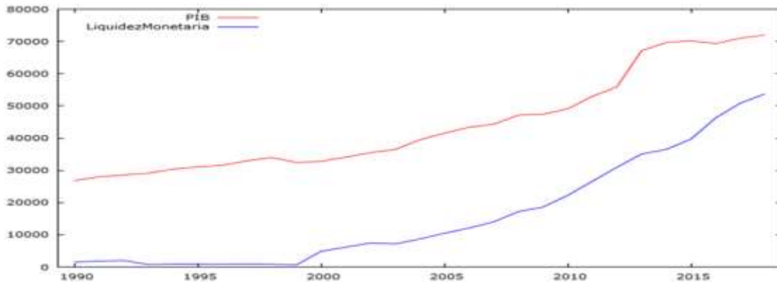
Fig. 14. Mínimos Cuadrados Ordinarios del modelo
